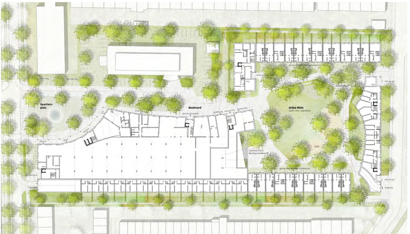
Lageplan
